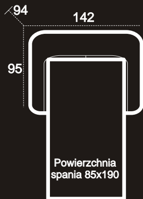
2R (kanapa 2-os.rozkładana stela RINO)
