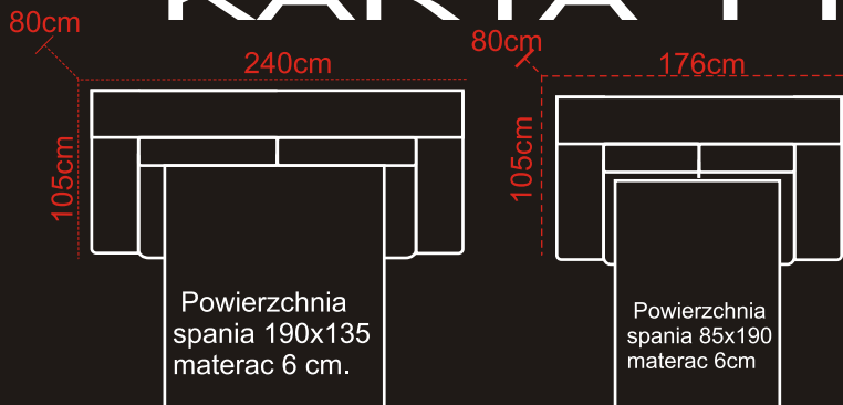
2R (kanapa 2-os.rozkładana stelaż RINO)
