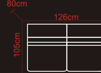
2-0 (kanapa 2-osobowa bez poręczy)
